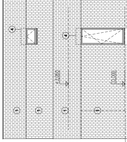
BOČNÍ(ZADNÍ) POHLED
